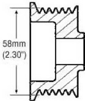
APS Part# F658 6 groove 58mm
