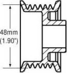
APS Part# F648 6 groove 48mm
