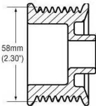
APS Part# F858 8 Groove 58mm
