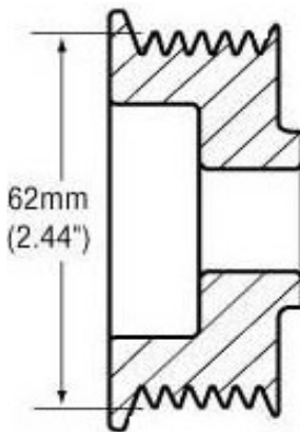
APS Part# G662 6 Groove 62mm
