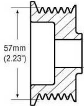
APS Part# G657 6 Groove 57mm
