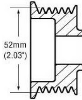
APS Part# G652 6 Groove 52mm
